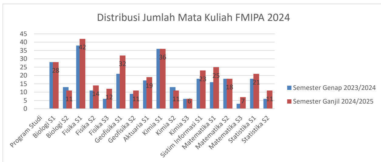
Gambar 1. Distribusi Jumlah Mata Kuliah Pada Tahun 2024 di FMIPA
